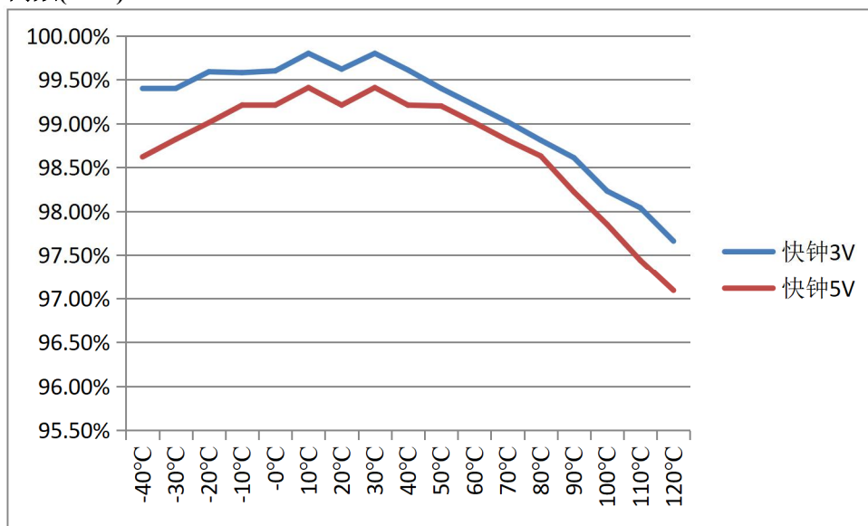
高频(16M)
