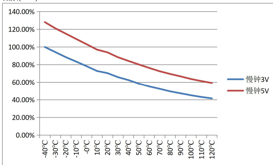
低频(32K)
